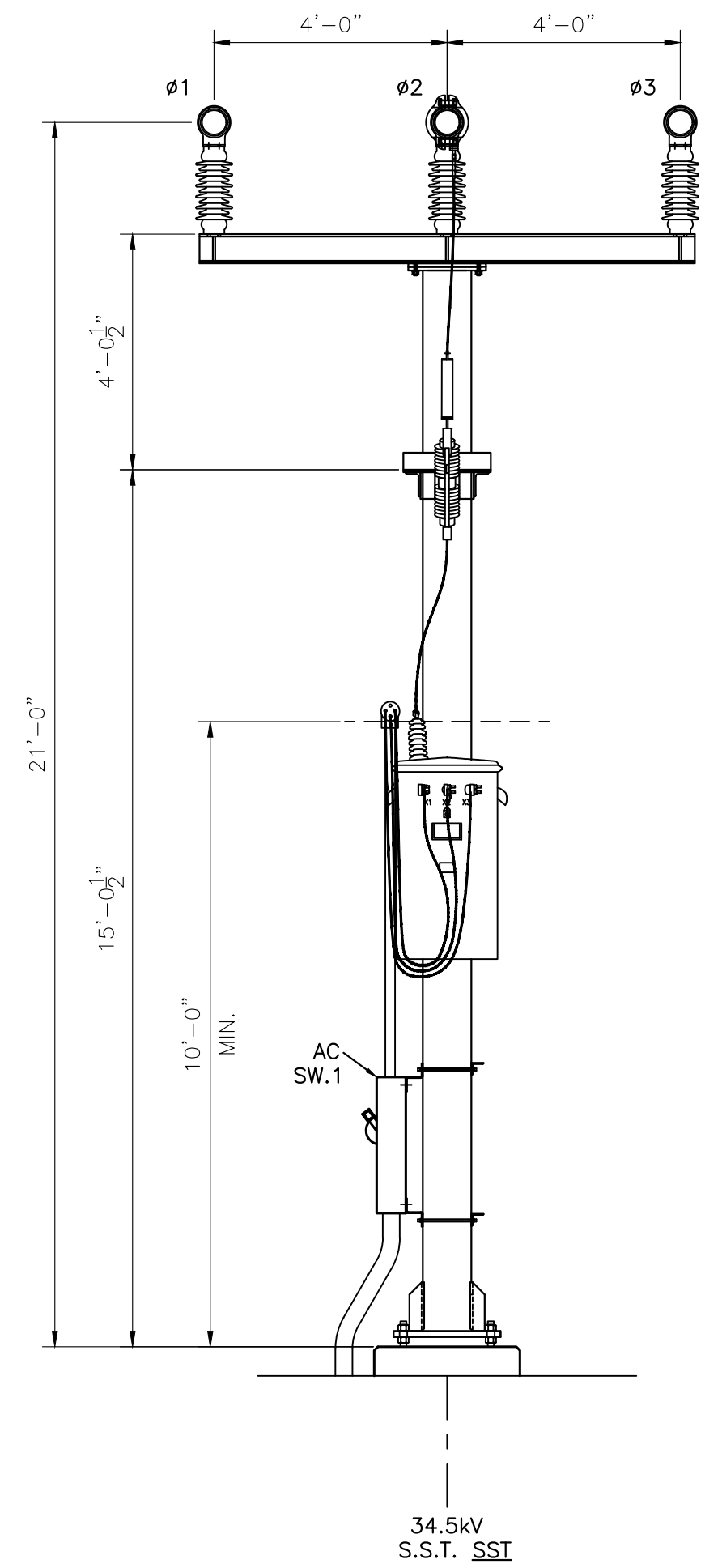
ELEVATION C-C
