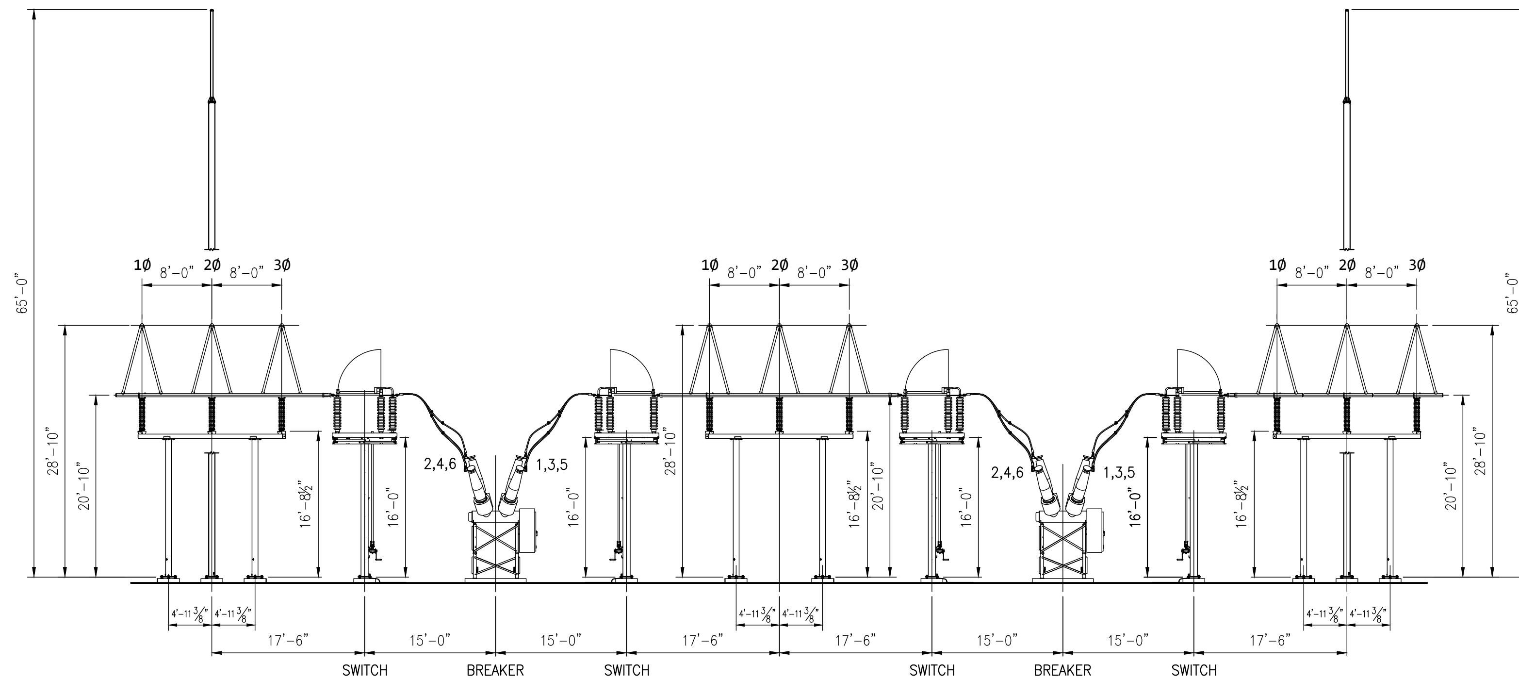
ELEVATION D-D
