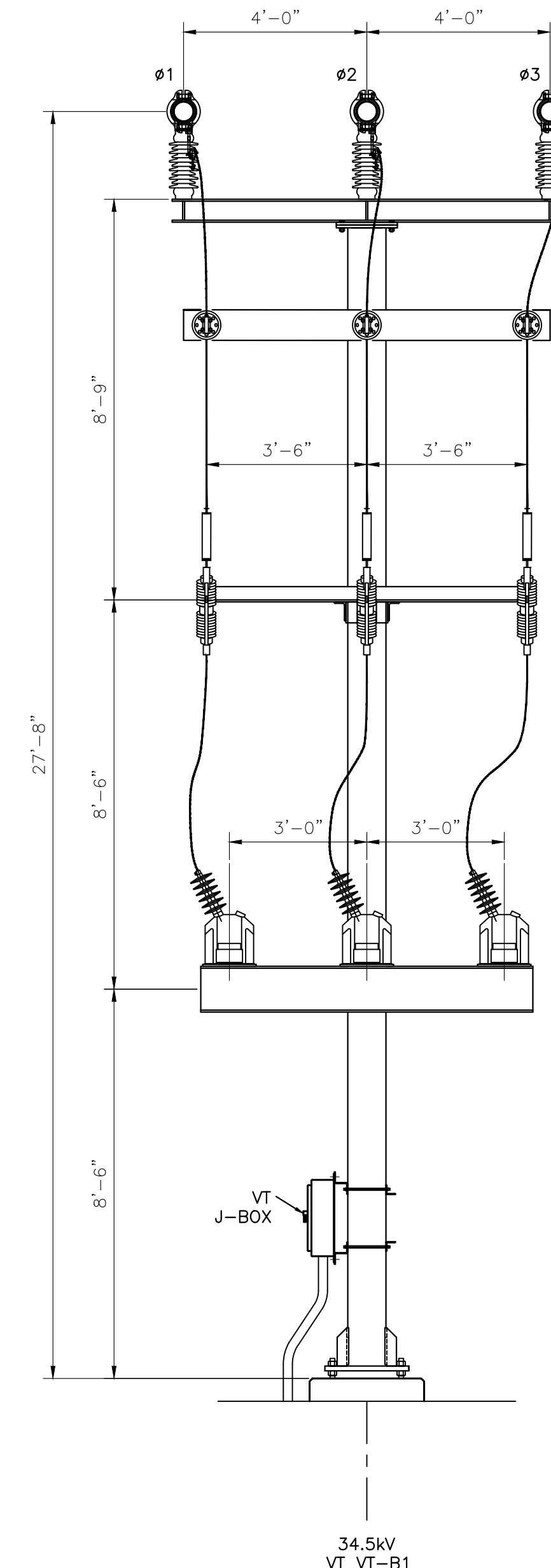
ELEVATION D-D
