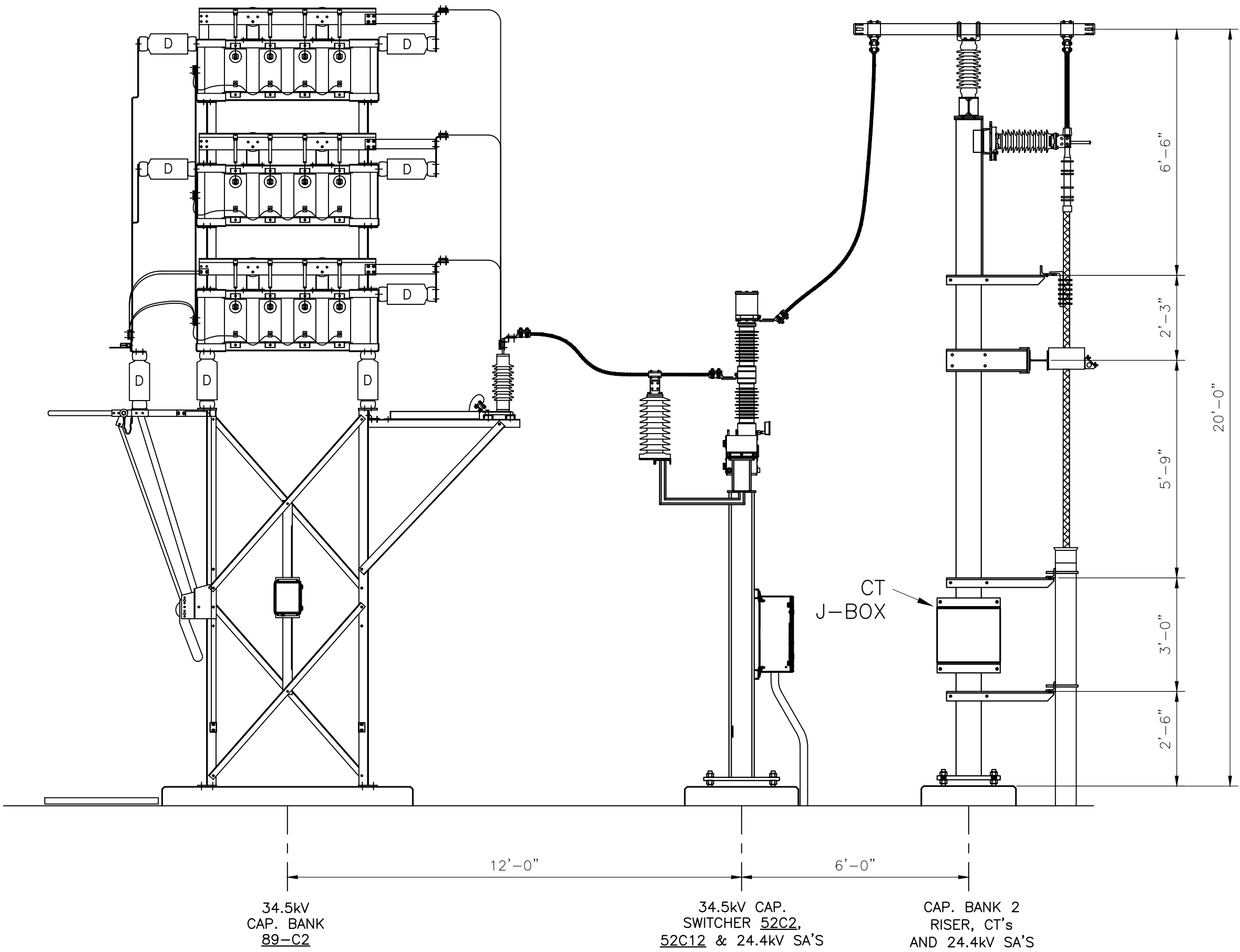
ELEVATION M-M
