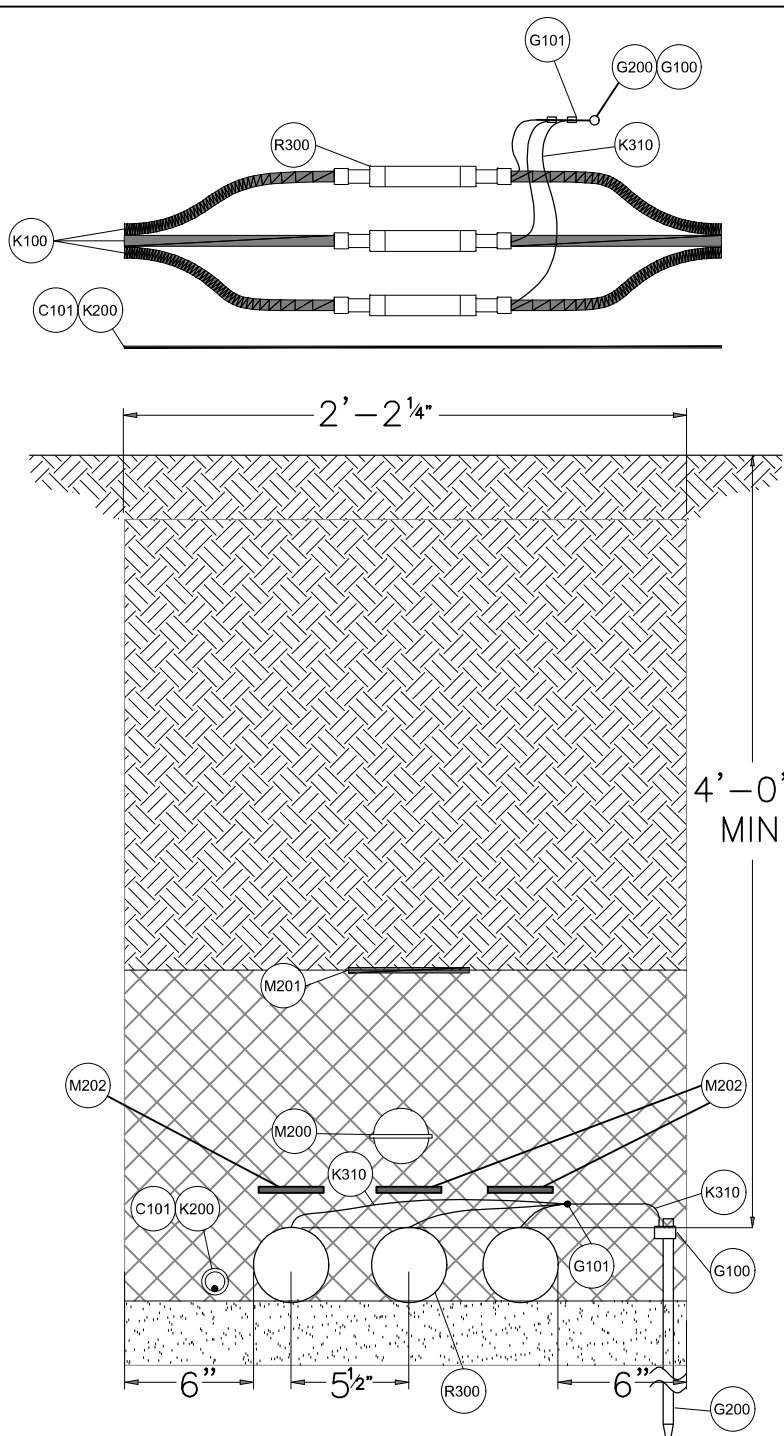
3 MV CABLE SPLICE DETAIL SCALE: N.T.S.
