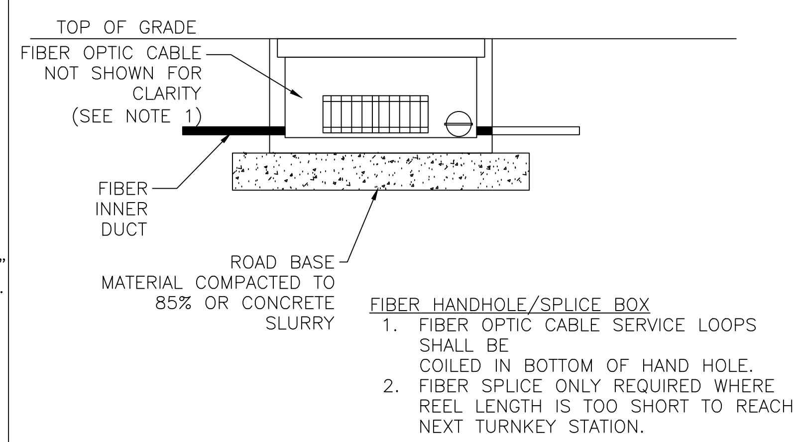
4 FIBER HANDHOLE/SPLICE BOX SCALE: N.T.S.
