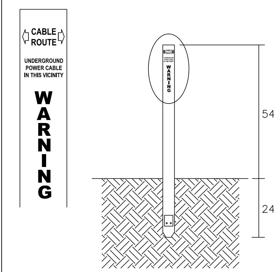
5 CABLE MARKER DETAIL SCALE: N.T.S.
